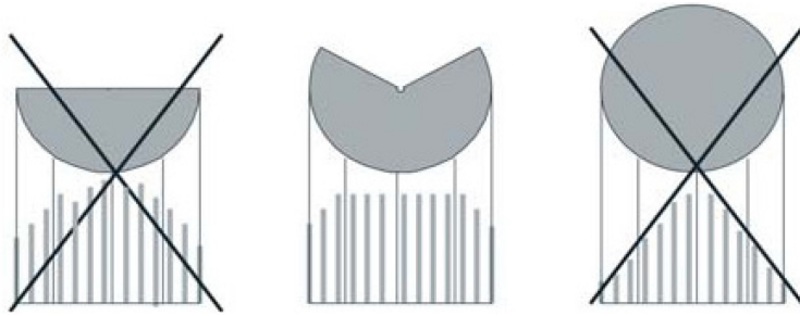
Figuur 11.4 De gewenste sectorinstelling voor een haspelinstallatie. De hoek is 240 graden. Met deze instelling wordt het beste sproeibeeld verkregen. De waternverdeling wordt aangegeven met de grijze balkjes.
