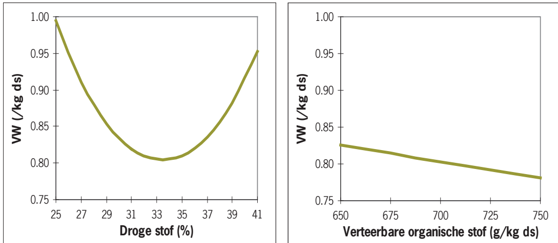
Figuur 12.1 Links de relatie tussen drogestofgehalte (%) en verzadigingswaarde bij een VOS-gehalte van 700g/kg ds; Rechts de relatie tussen het VOS-gehalte (g/kg ds) en de verzadigingswaarde bij een drogestofgehalte van 33%
